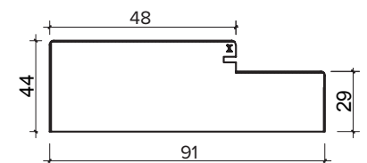
ASTRAGAL
